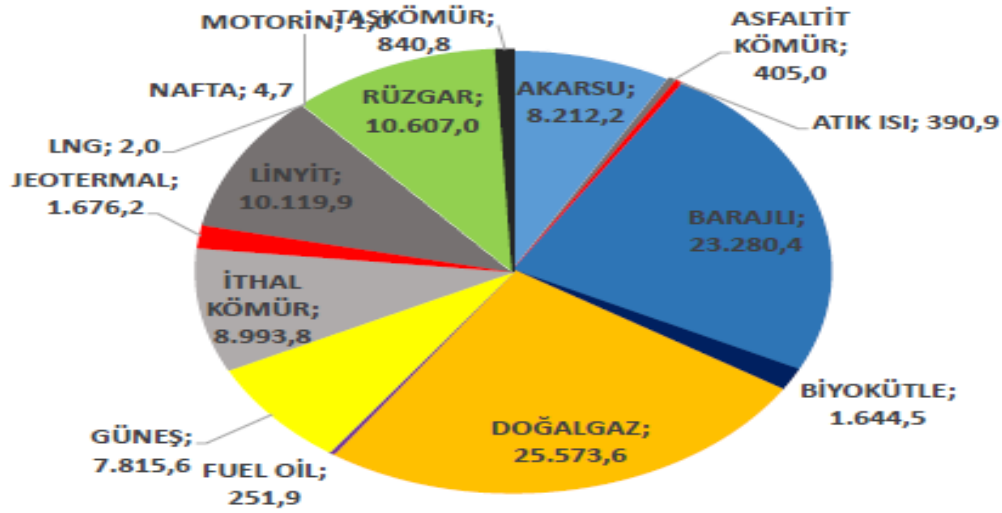
Şekil 6-Türkiye’de elektrik kurulu gücünün kaynaklara göre dağılımı –Aralık 2021 Kaynak: TEİAŞ
